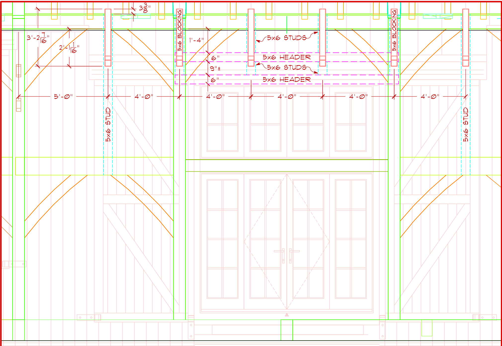
WALL 4 ELEVATION Scale: \frac{3}{8}'' = 1'-0''
